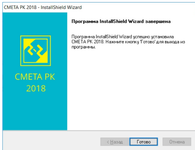
Рис.6. Завершение установки
