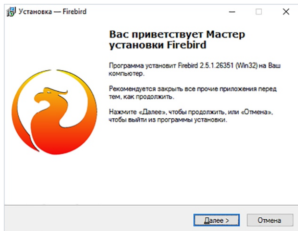
Рис.5. Установка Firebird
